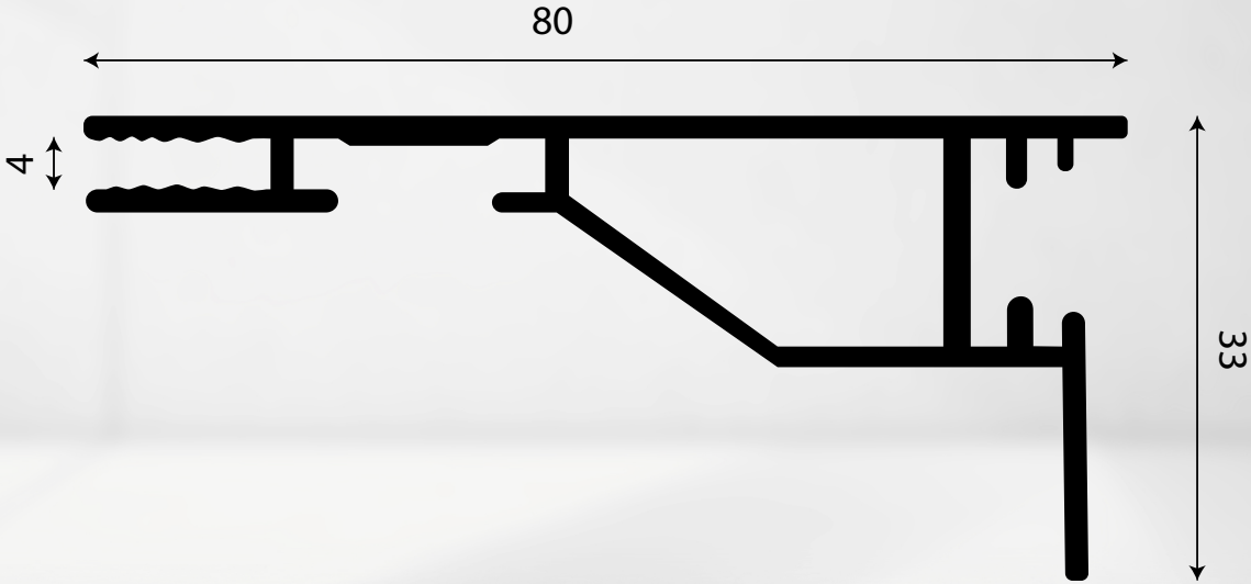
Mặt cắt ngang Horizontal section
